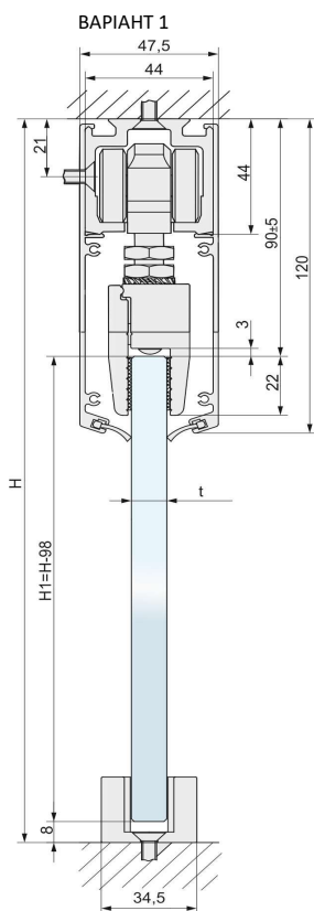
Рухоме дверне полотно
