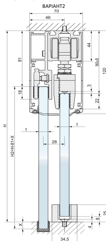
Дверне полотно з фіксованим склом
