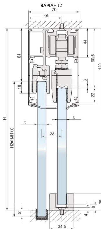
Дверне полотно з фіксованим склом
